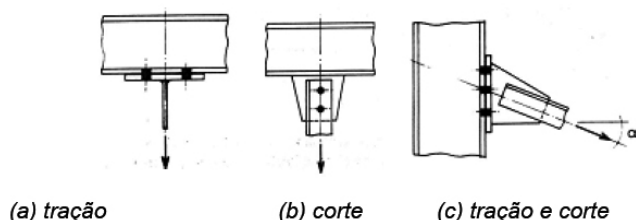
Figura 15 - Conexões por contato.
