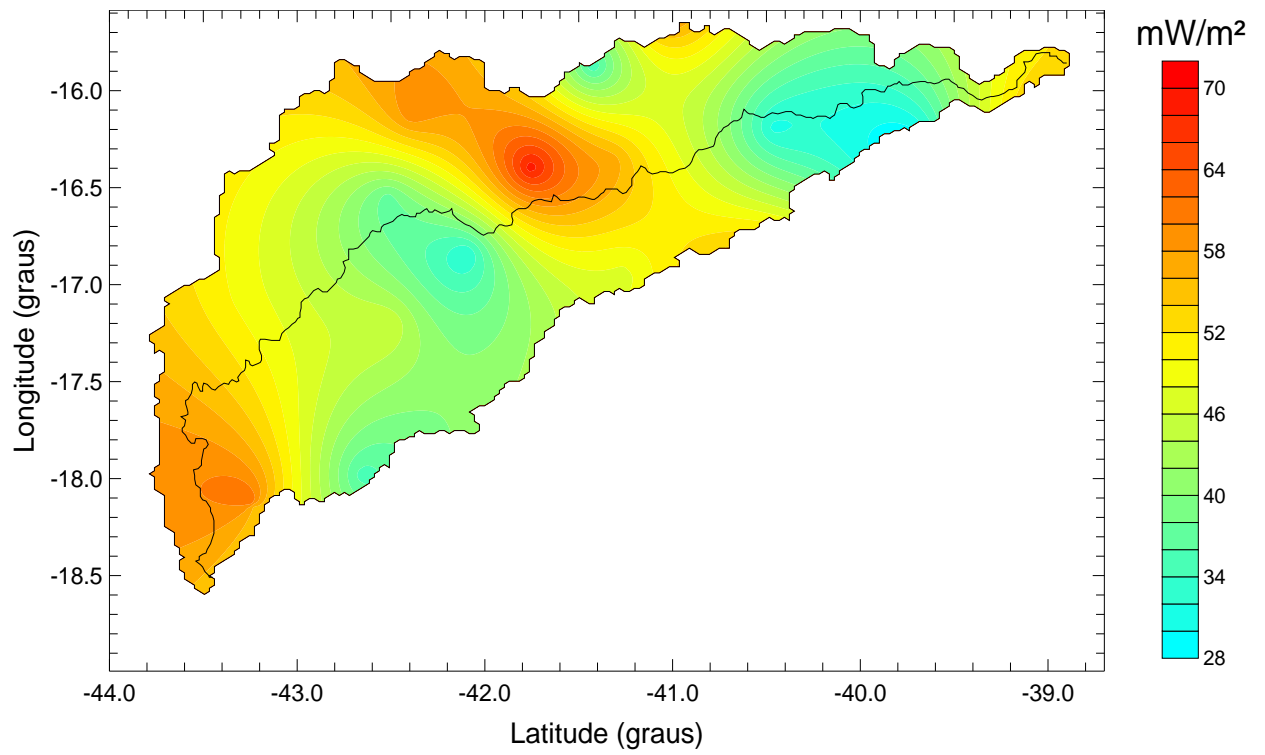
Mapa da Distribuição do Fluxo de Calor Geotérmico na Bacia do rio Jequitinhonha
