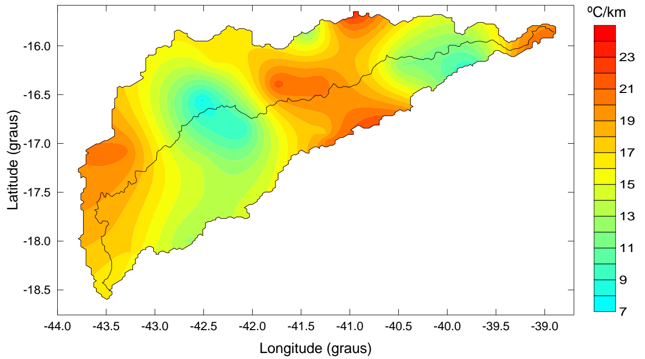
Mapa da Distribuição do Gradiente Geotérmico na Bacia do rio Jequitinhonha
